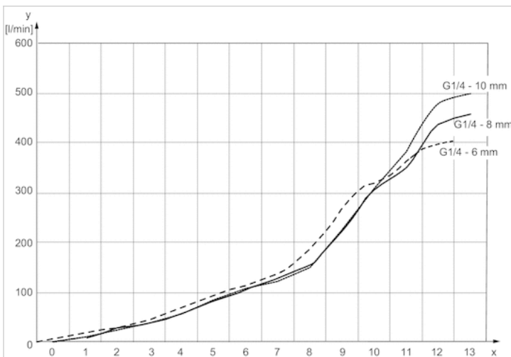
Durchflussdiagramm Fig. 3
